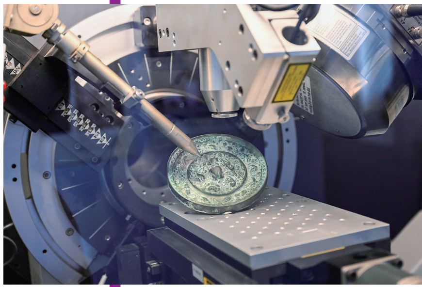
这是展出的二维面探测器X射线衍射仪。新华社记者 金良快 摄
