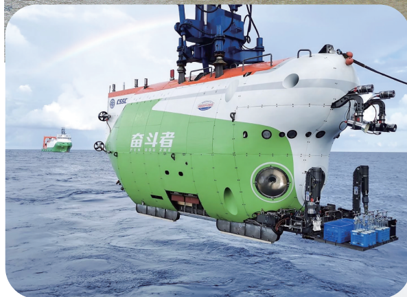
▲“奋斗者”号(资料照片)。 新华社发(中国船舶集团供图)
