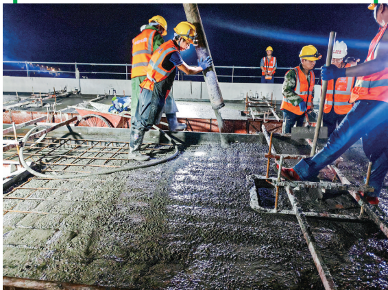
袂花江特大桥无砟轨道底座板混凝土浇筑施工。 通讯员武聚盟 摄
