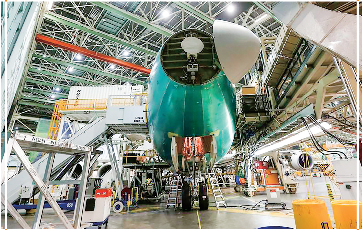
这是波音埃弗里特工厂747飞机生产线上正在组装的747-8飞机(2014年9月29日摄)。新华社记者张玉薇摄
