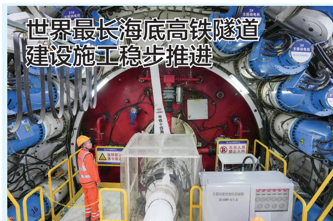
2月11日,中铁十四局技术人员在甬舟铁路金塘海底隧道“甬舟号”盾构机内关注设备运行情况。
