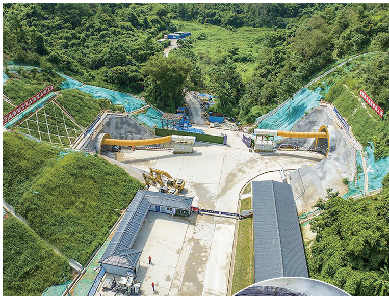
环北部湾供水项目(高州大井段)。本报记者 甘杨松 摄
